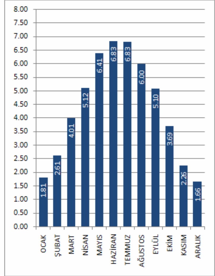
MUŞ İLİ GLOBAL RADYASYON DEĞERLERİ (KWh/m 2 -gün)
