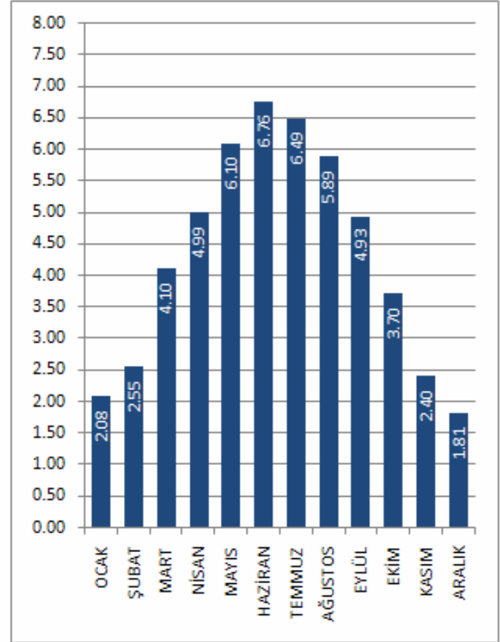
KİLİS İLİ GLOBAL RADYASYON DEĞERLERİ (KWh/m 2 -gün)
