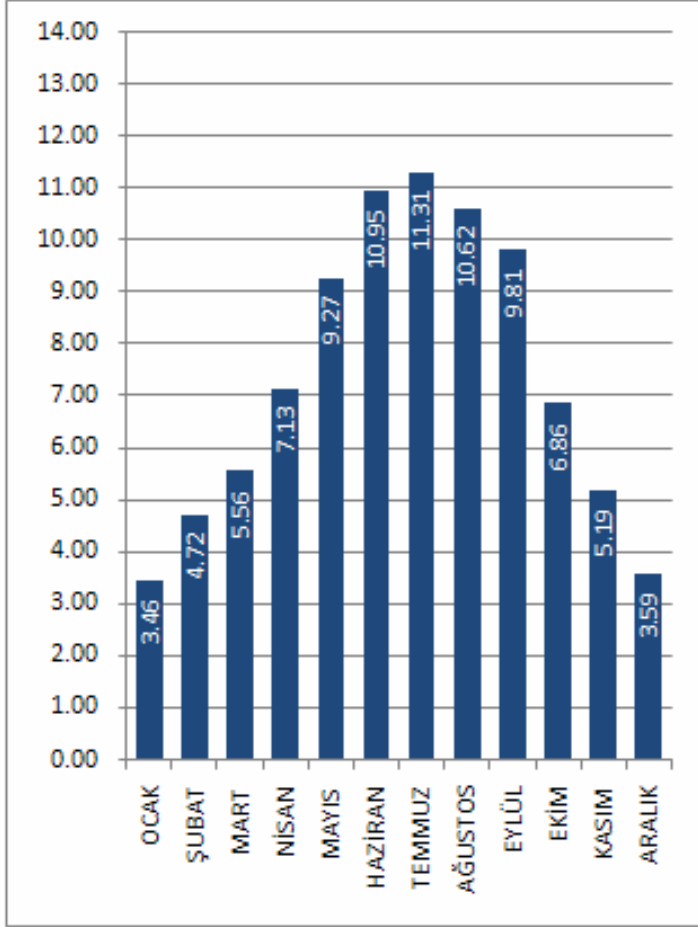
BİTLİS İLİ GÜNEŞLENME SÜRESİ DEĞERLERİ (Saat)
