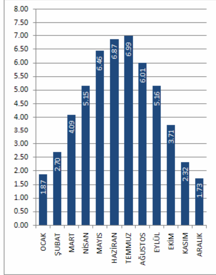
BİTLİS İLİ GLOBAL RADYASYON DEĞERLERİ (KWh/m 2 -gün)
