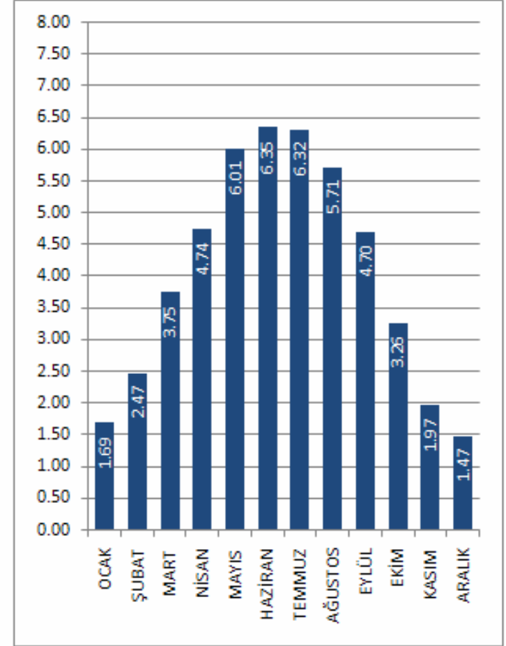
ANKARA İLİ GLOBAL RADYASYON DEĞERLERİ (KWh/m 2 -gün)
